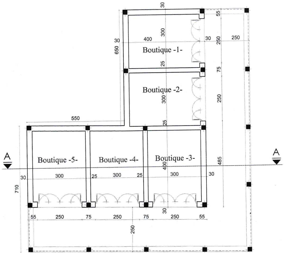
PLAN REZ DE CHAUSSEE
